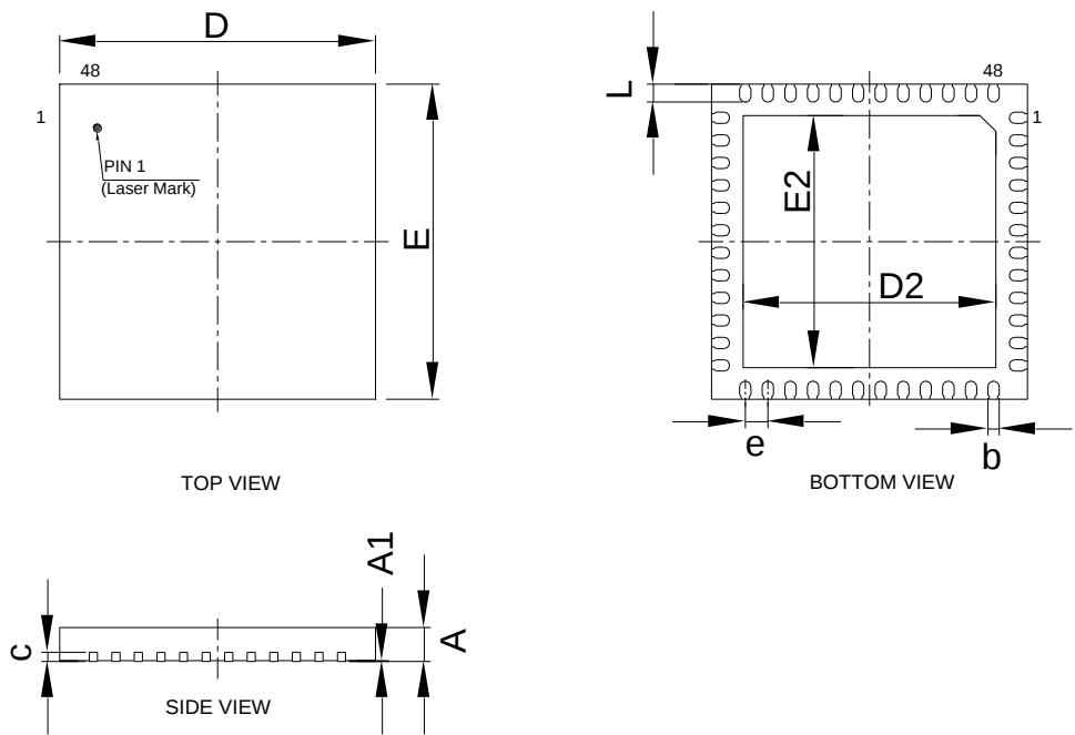
图 19 QFN48 封装图
