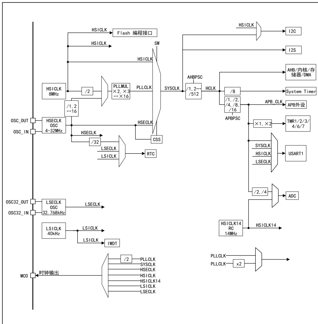
图 6 时钟树
