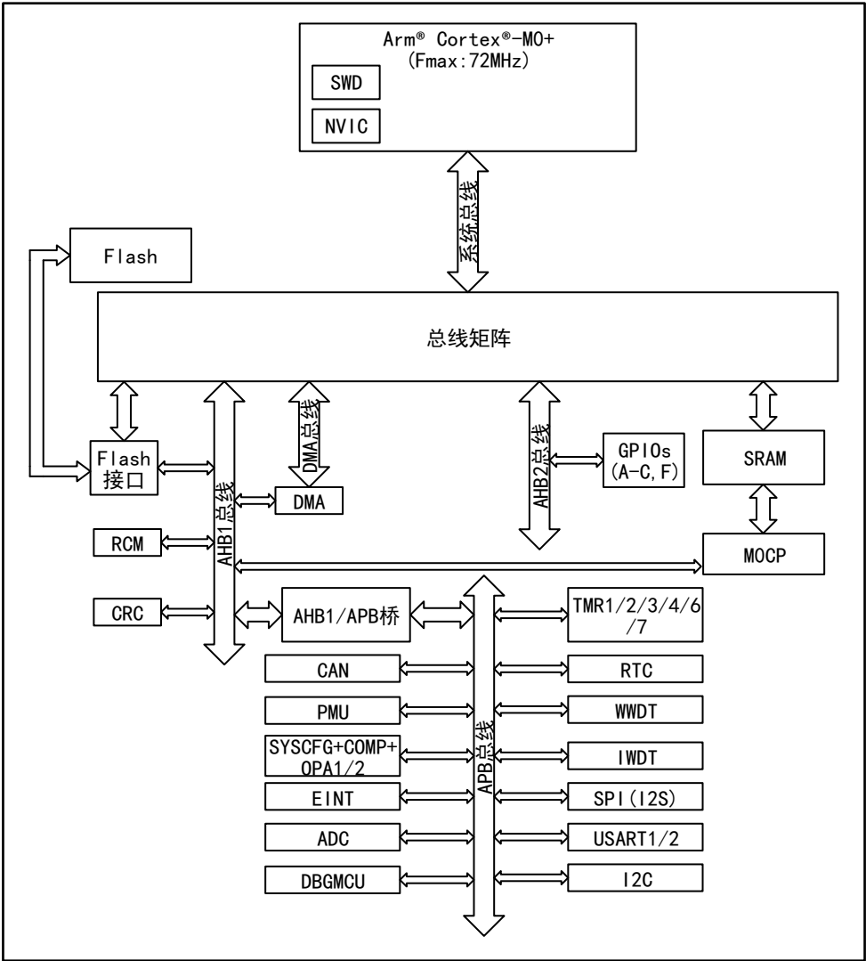
图 4 APM32F035x8 产品系统框图
