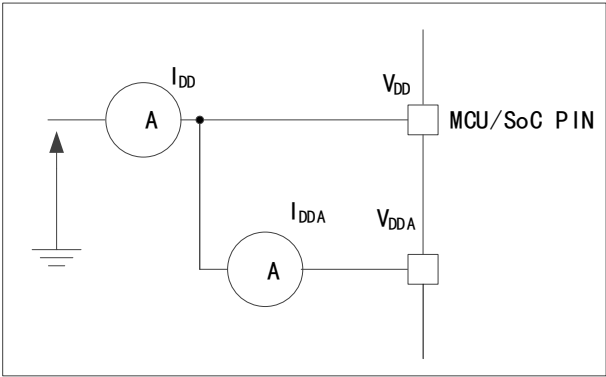
图 10 电流消耗测量方案
