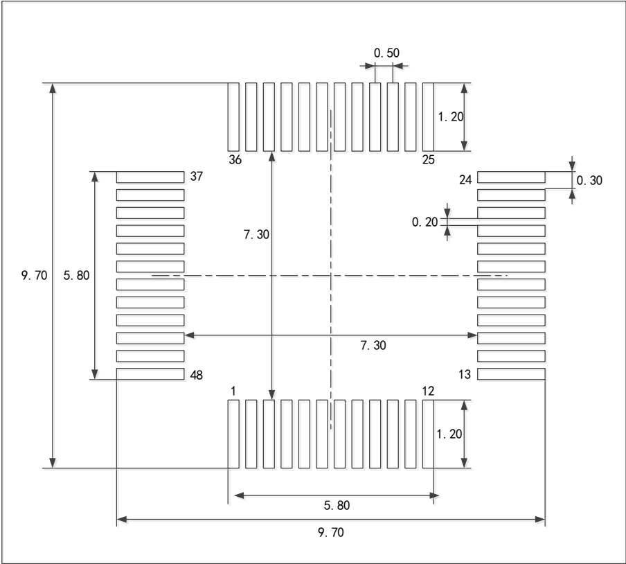
图 18 LQFP 焊接 Layout 建议
