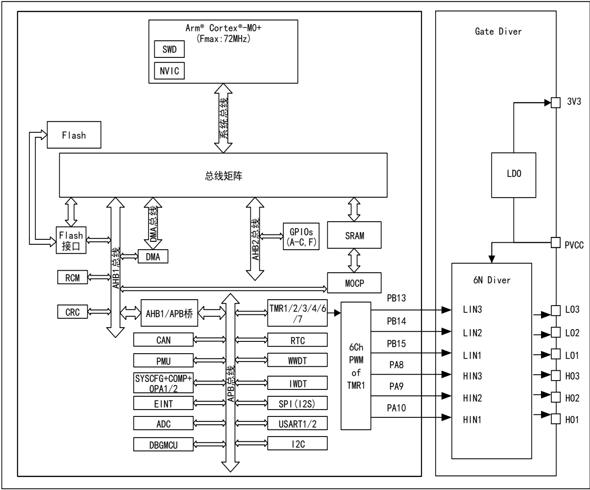
图 5 APM32M3514x8 产品系统框图
