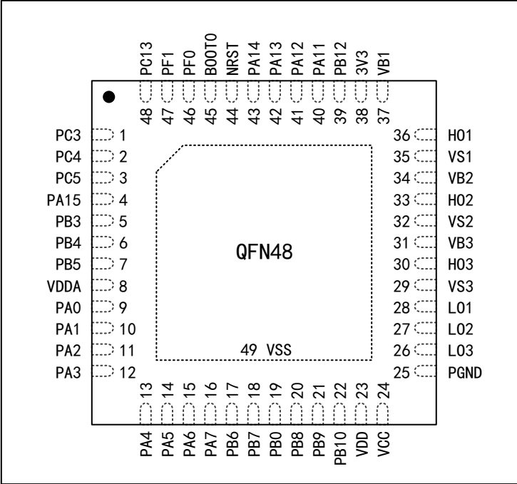
图 3 APM32M3514x8 产品 QFN48 引脚配置图
