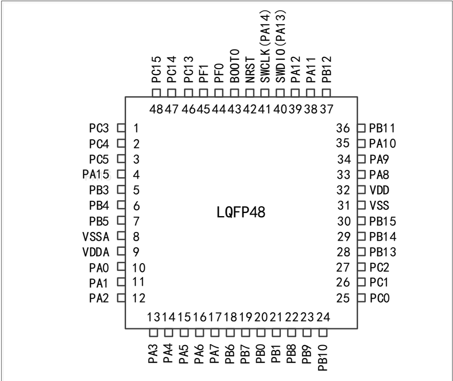
图 1 APM32F035x8 产品 LQFP48 引脚配置图
