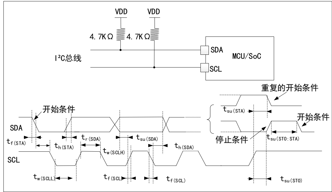
图 12 总线交流波形和测量电路
