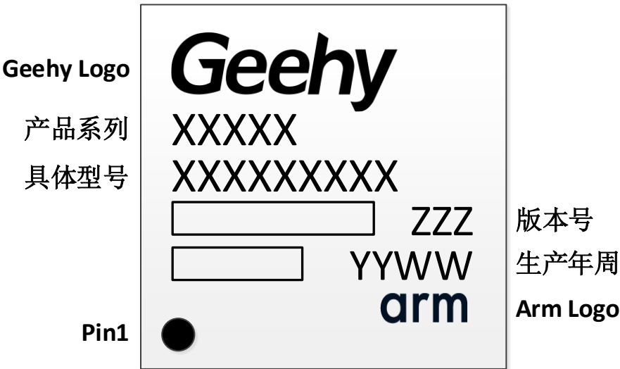
图 16 产品丝印图
