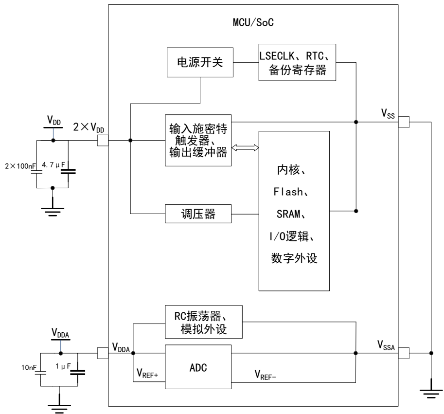
图 7 电源方案
