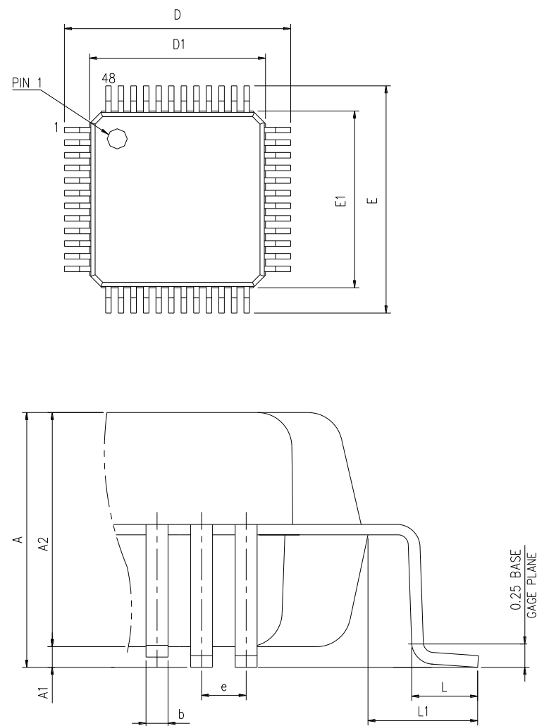
图 17 LQFP48 封装图
